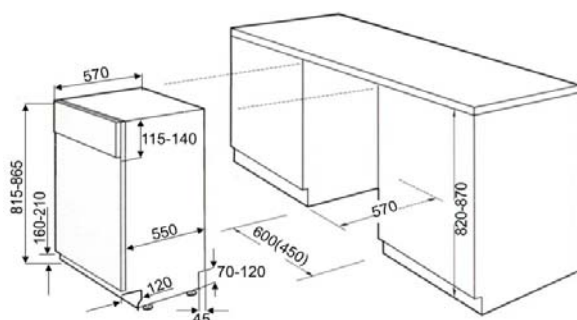
Einbauskeizze
