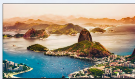
H.265 HEVC
