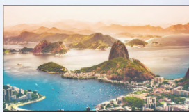
H.264
