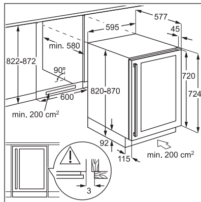
Installasjonsdiagram for kvalifisert montør.
