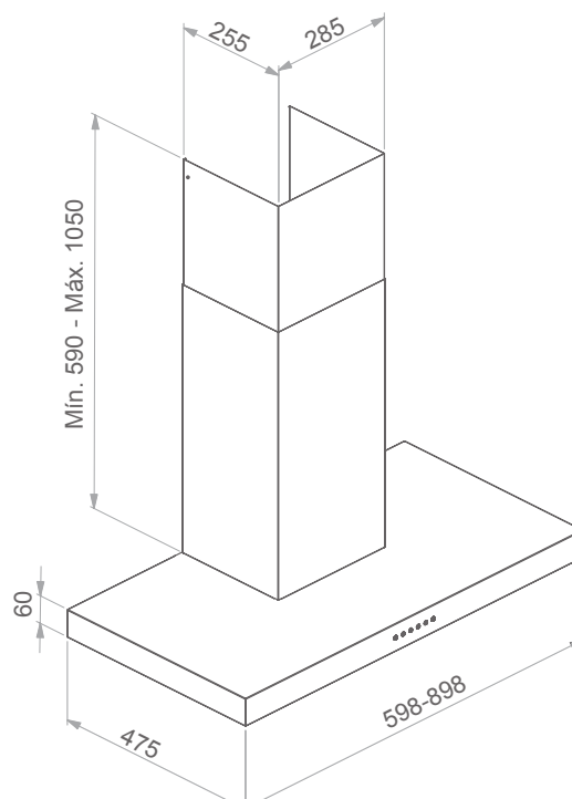
Medidas en mm Tubos regulables en altura
