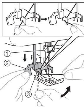
① Nadelhalter ② Nadeleinfädlerhebel ③ Führung
