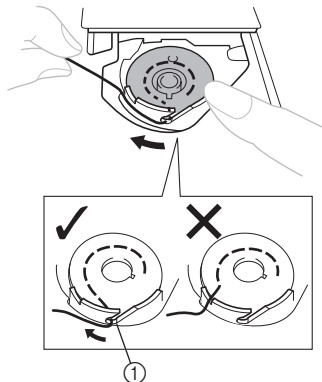
① Spannungseinstellfeder
