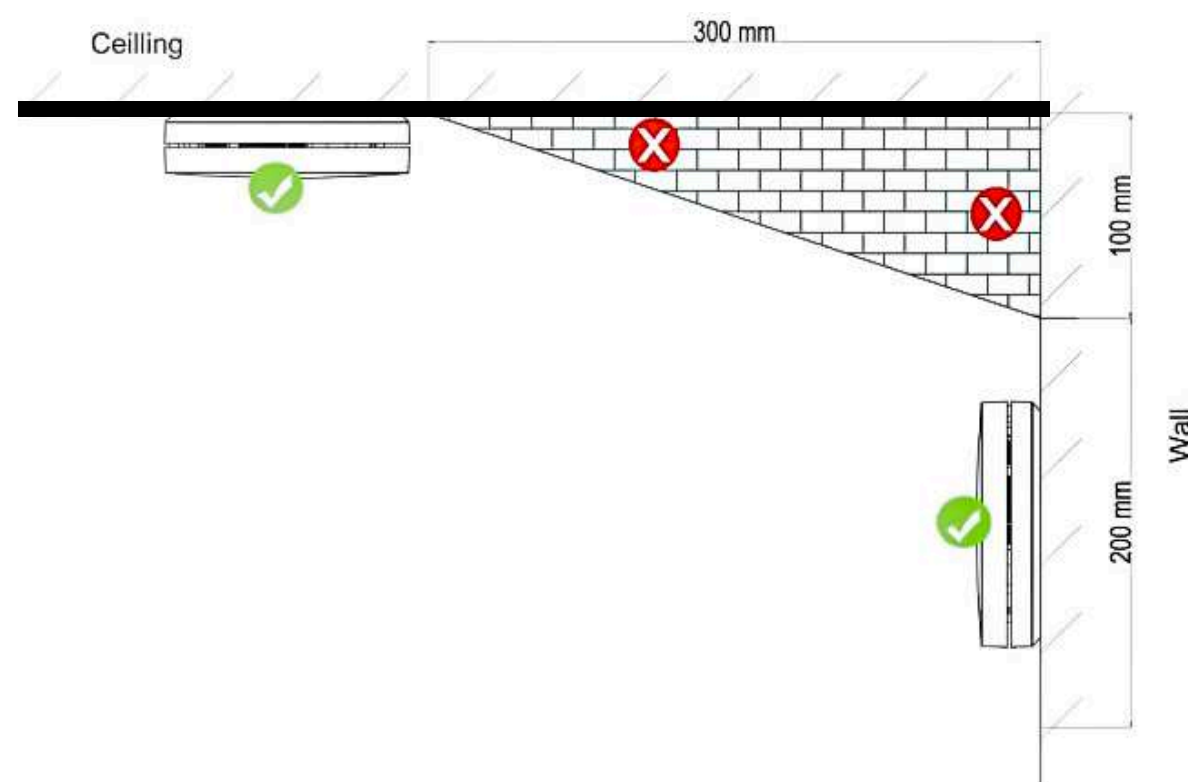
Figura 3: posizioni di montaggio consigliate
