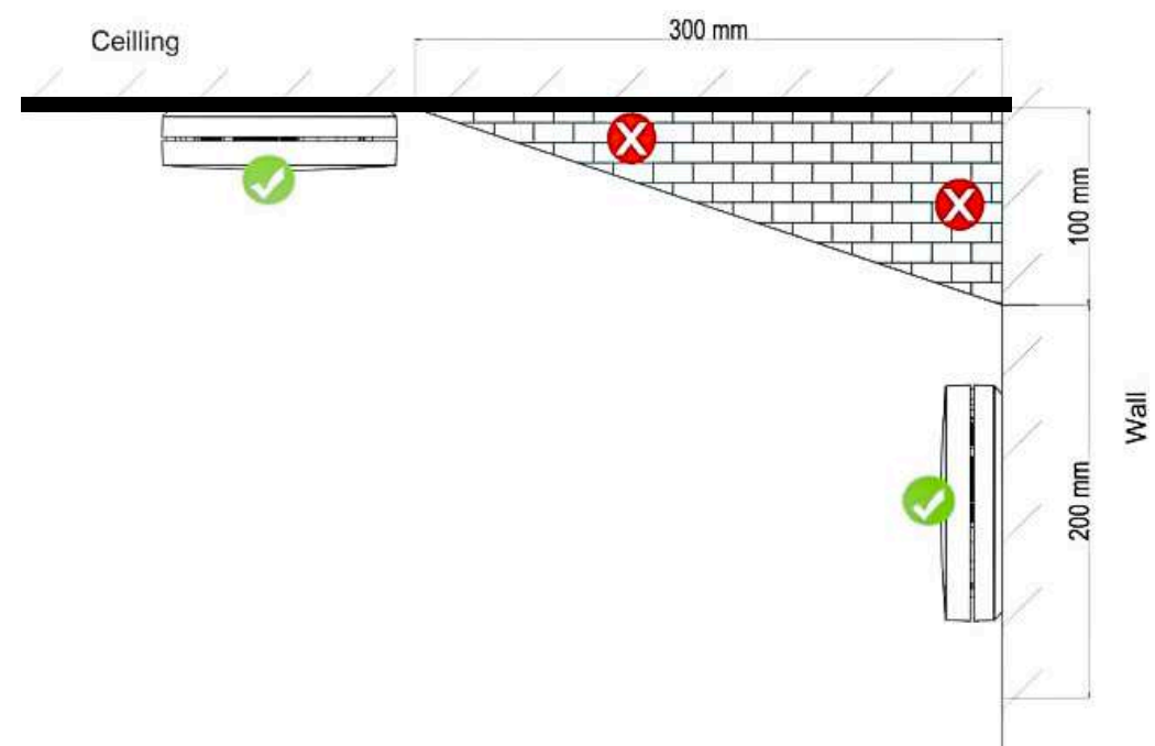
Abbildung 3: Empfohlene Montageorte
