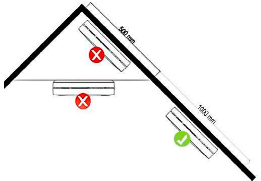
Abbildung 2: Empfohlene Montageorte
