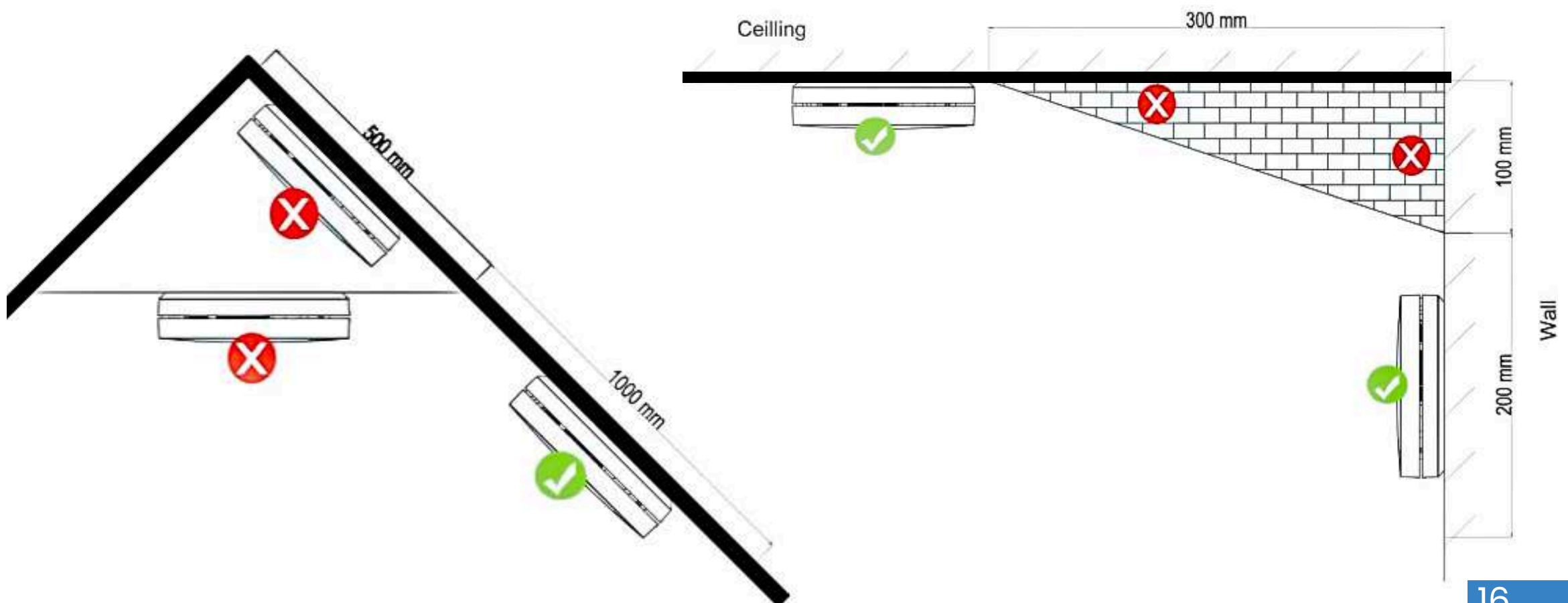
Figure 4 : Emplacements de montage recommandés
