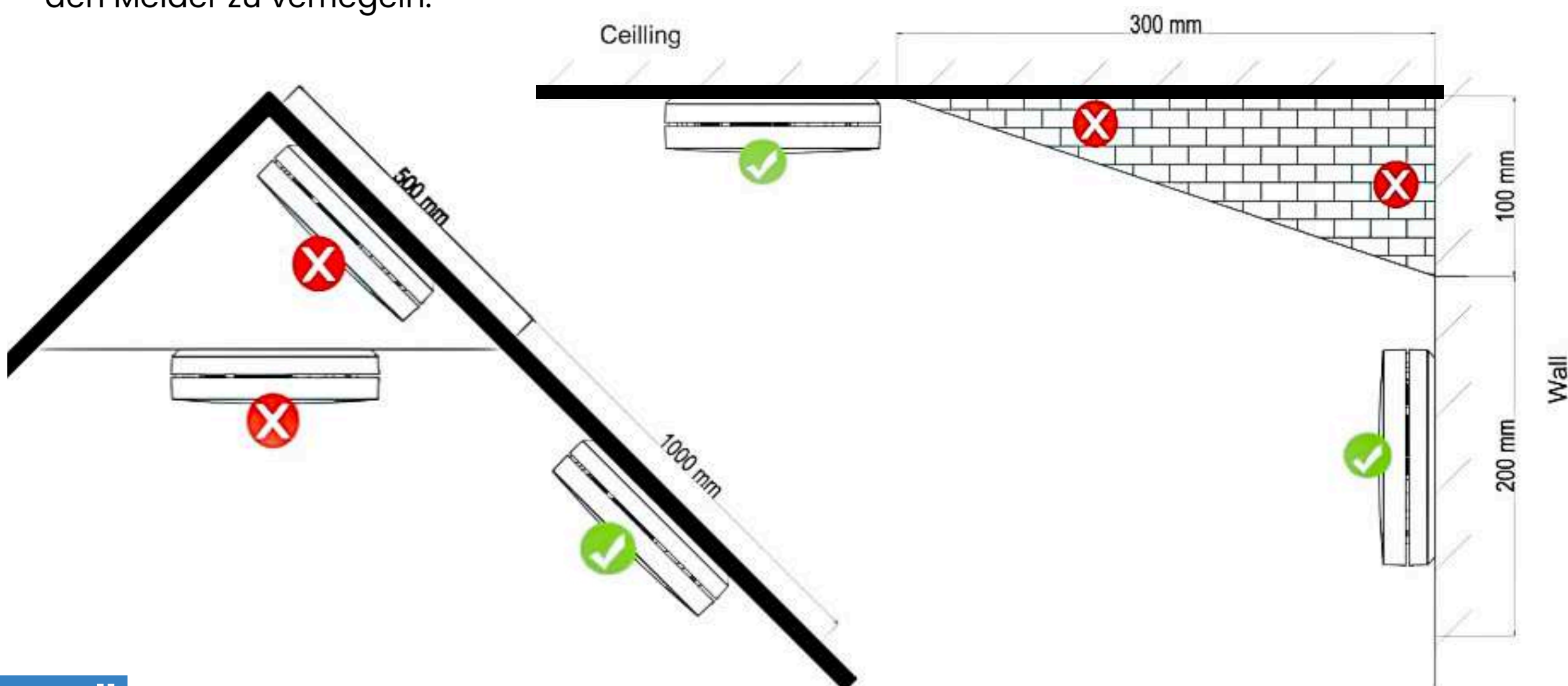
Abbildung 4: Empfohlene Montageorte
