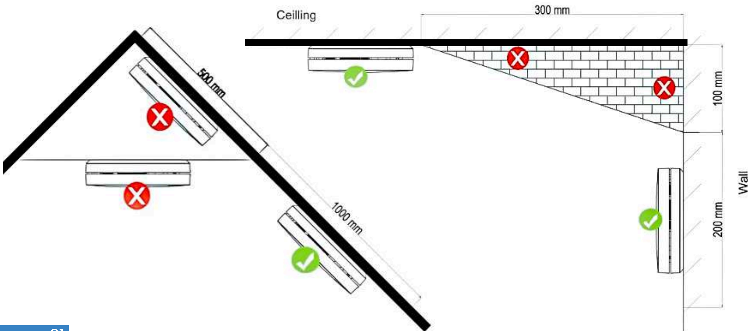
Figura 5: Ubicaciones de montaje recomendadas
