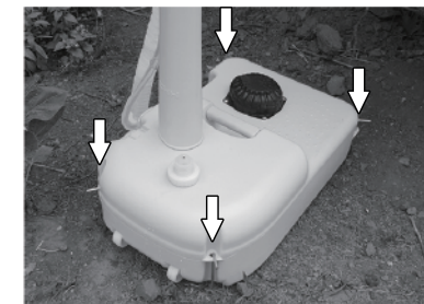
El tanque de base puede ser fijado en el suelo a través de cuatro agujeros en la esquina si es necesario
