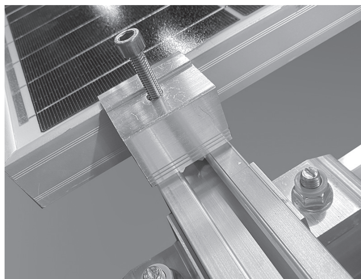
Modulendhalter
