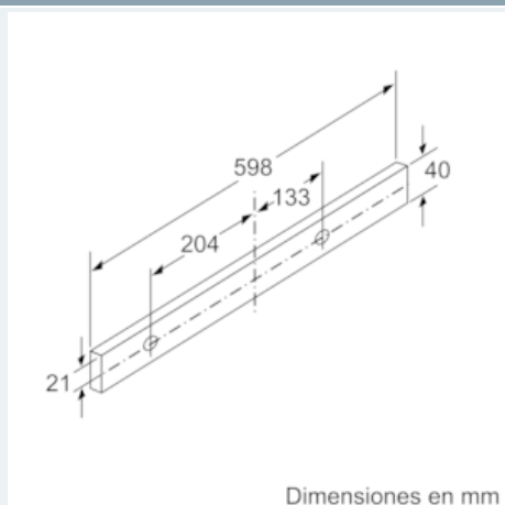
Dibujos acotados
