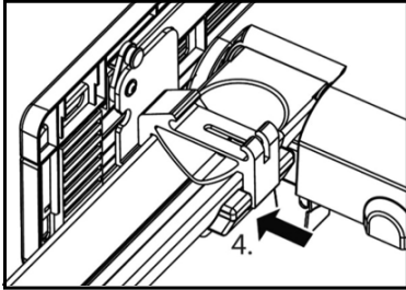
Bild 6: Montage Aluminiumadapter
