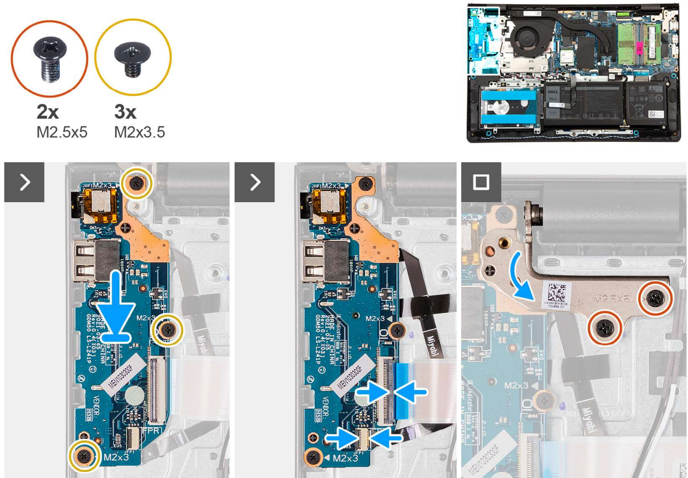
Abbildung 7. Einbauen der I/O-Tochterplatine
