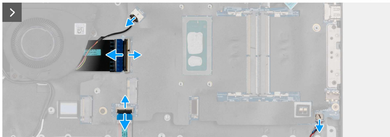
Abbildung 58. Entfernen der Systemplatine
