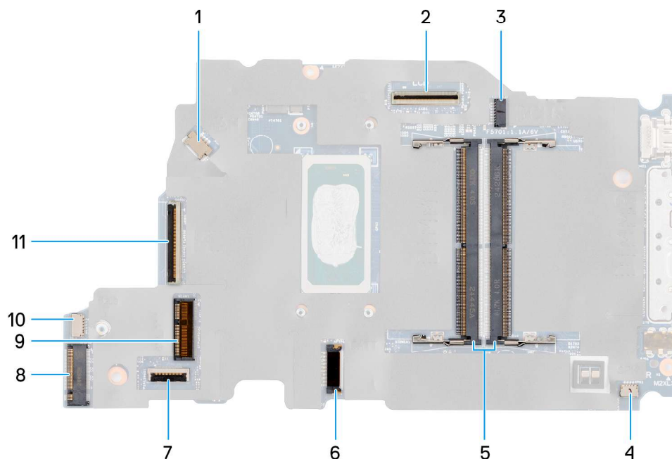
Abbildung 63. Hauptplattenanschlüsse
