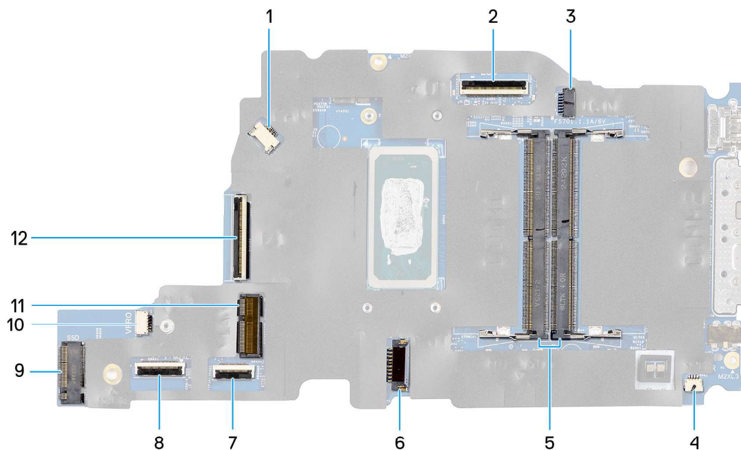
Abbildung 69. Hauptplattenanschlüsse
