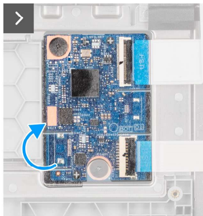
Abbildung 37. Entfernen der USH-Platine
