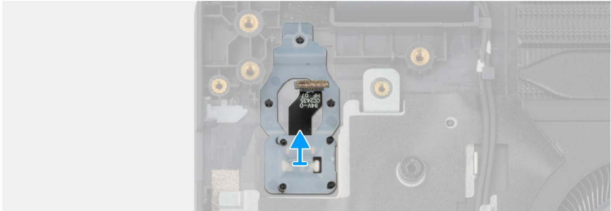
Abbildung 55. Entfernen des Netzschalters mit Fingerabdruck-Lesegerät
