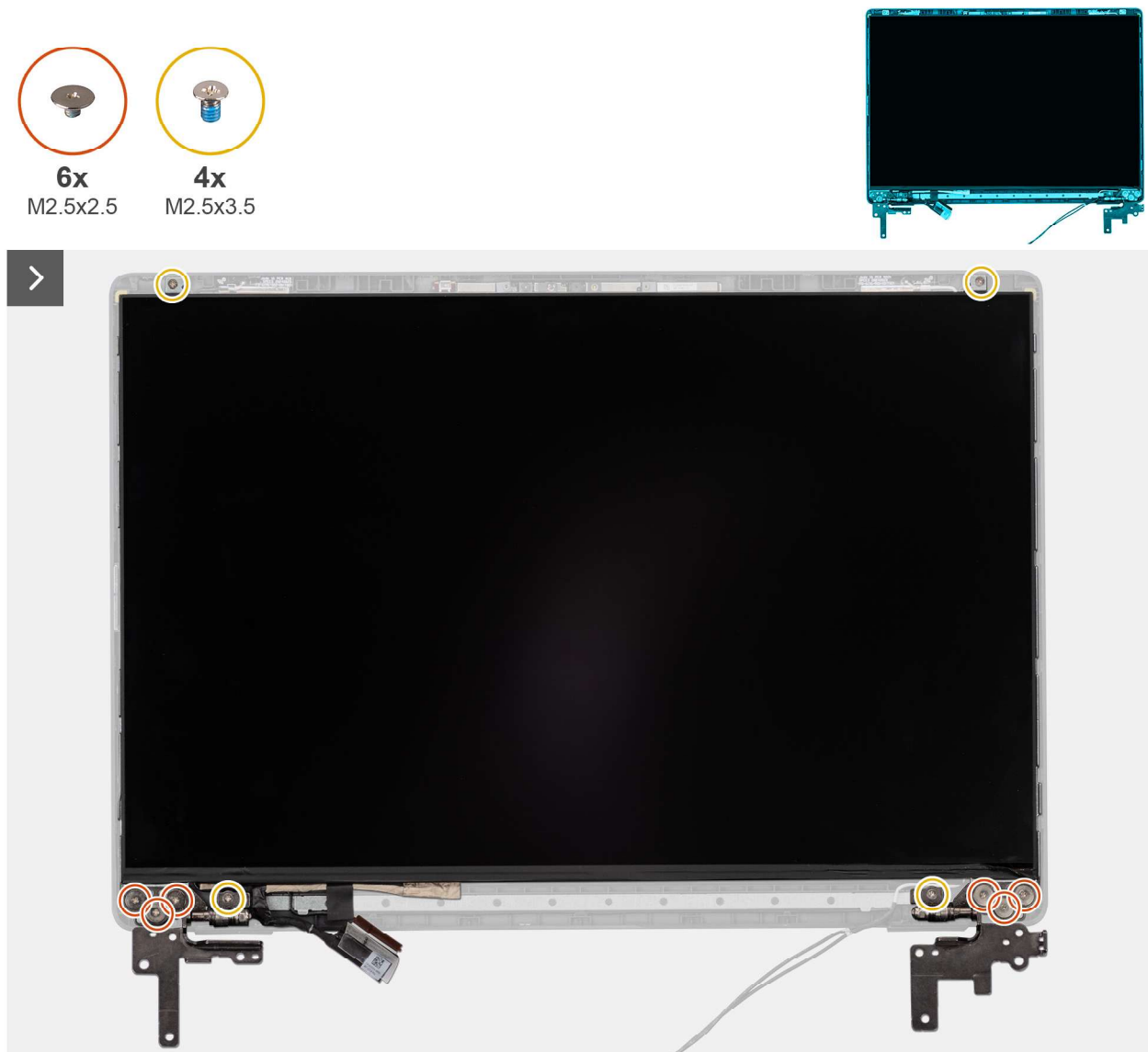
Abbildung 105. Entfernen der Bildschirmbaugruppe
