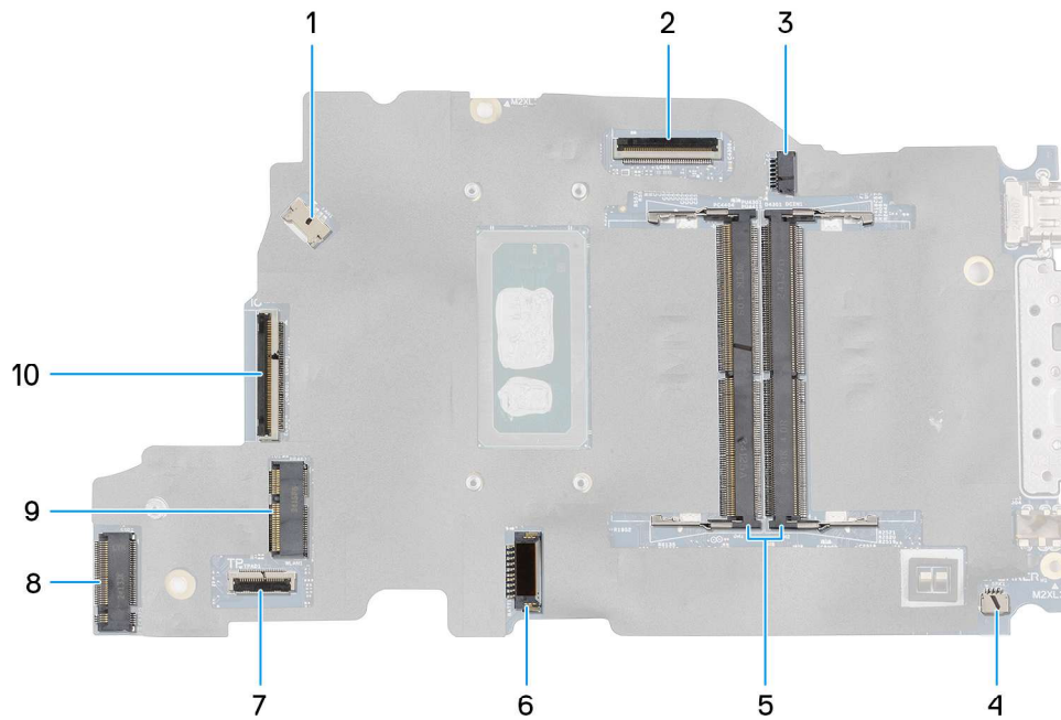
Abbildung 60. Hauptplatinenanschlüsse
