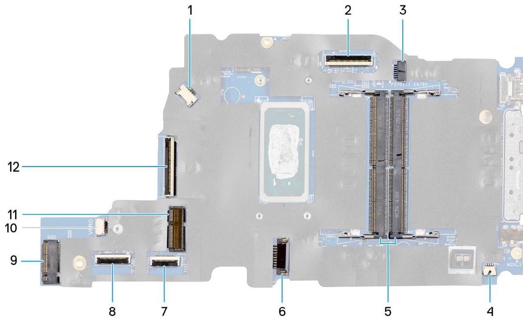
Abbildung 72. Hauptplatinenanschlüsse
