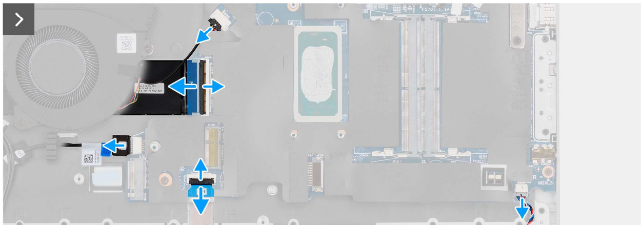
Abbildung 64. Entfernen der Systemplatine
