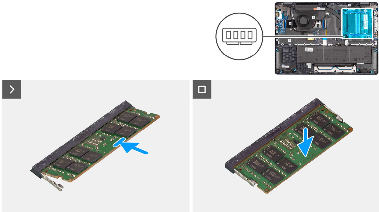
Abbildung 22. Einsetzen des Speichermoduls
