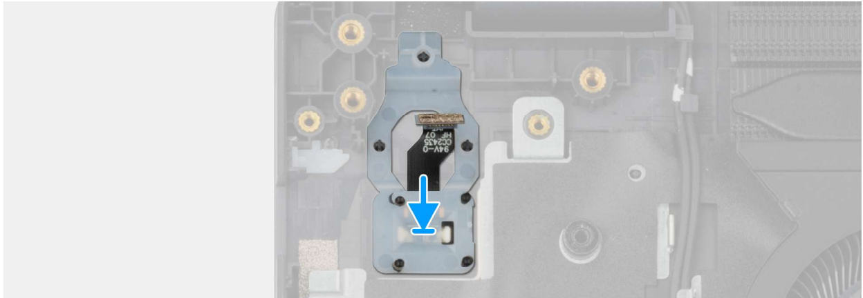
Abbildung 41. Einbauen des Netzschalters mit Fingerabdruck-Lesegerät
