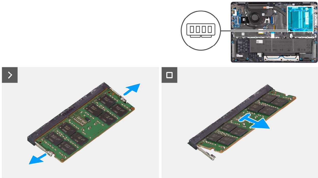
Abbildung 21. Entfernen des Arbeitsspeichersmoduls
