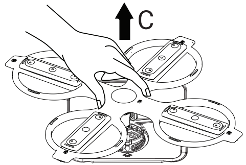
Darstellung 7.7: Entfernen des unteren Sprüharms
