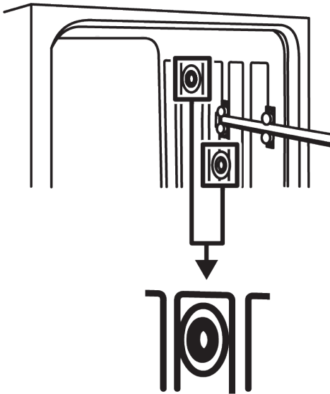
Abbildung 1 Fächertrocknungssystem
