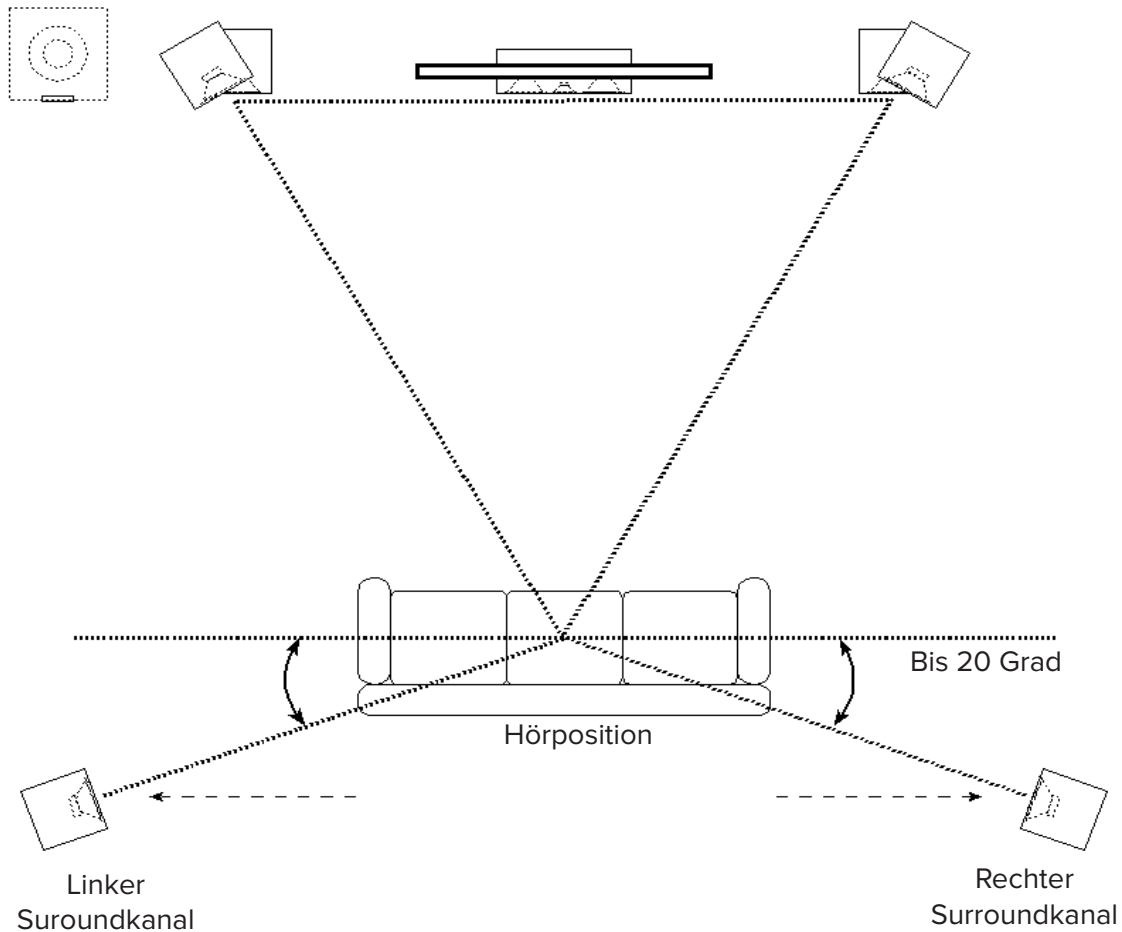
5.1-Kanal Surround Konfiguration
