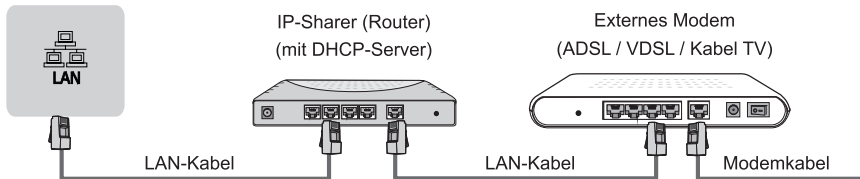
TV STECKBÜCHSE
