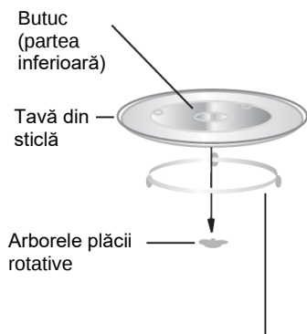
Ansamblu inel pentru placa rotativă
