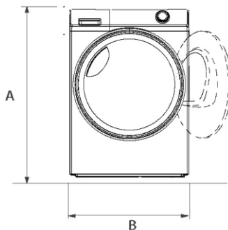
ELÖLNÉZET
