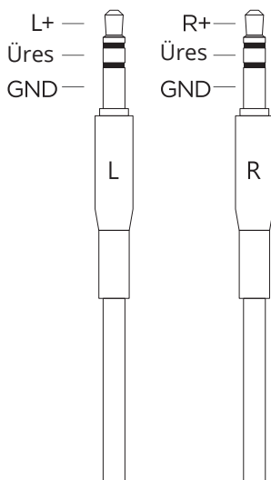
Kétoldalas 3,5 mm-es kábel
