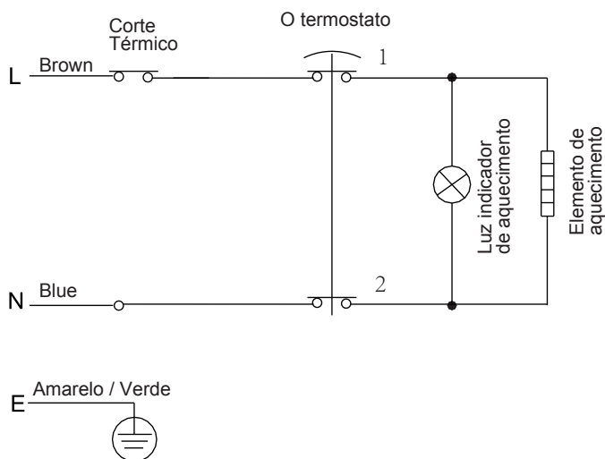
DIAGRAMA DE FIAÇÃO
