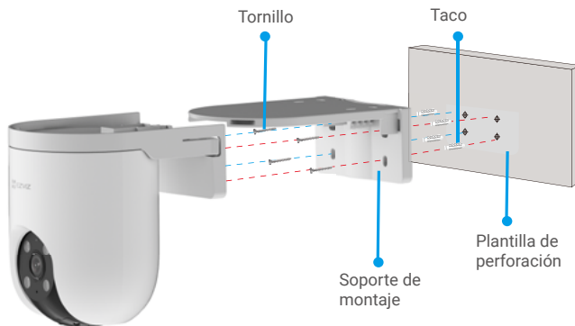
Figura 2. Montaje en pared
