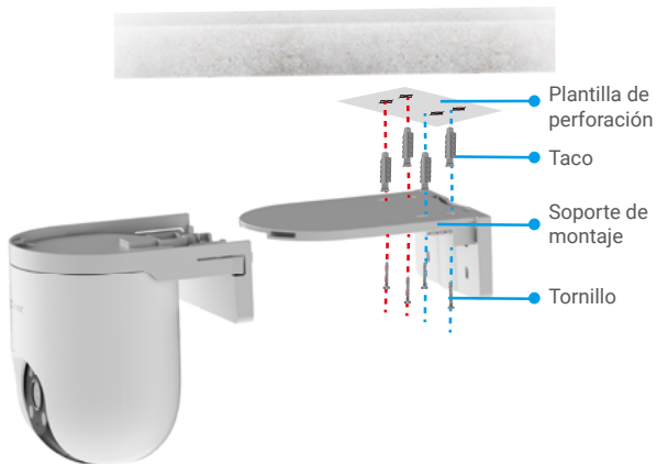
Figura 1. Montaje en techo
