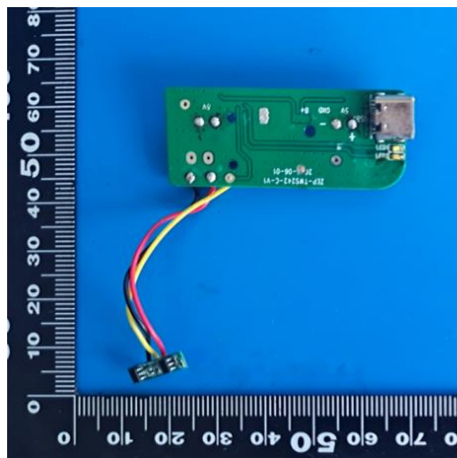
Fig. 6 – Back view of PCM 表6 – PCM 反面视图
